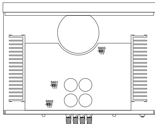
Jumper Locations Emplacement des Cavaliers Jumperposition Le posizioni dei ponticelli Ubicaciones de los Puentes
